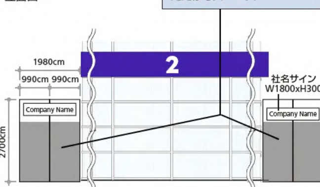
立面図
